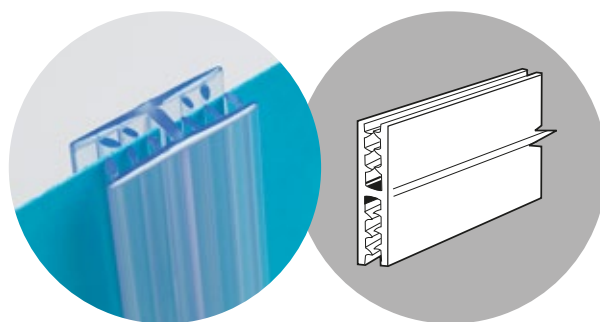
Grippeur d'assemblage en H Supergrip®
