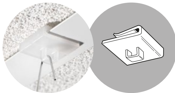
Crochet de suspension fermé
