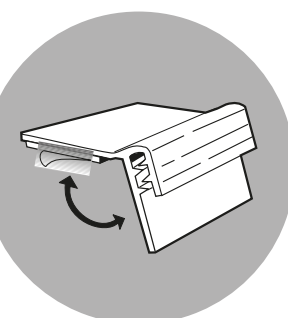
Support d'affichette articulé (à soulever) Supergrip®
